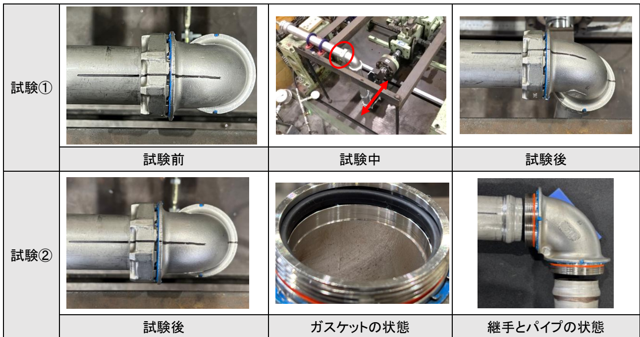
写真 4-15 揺動試験 I 試験後の状態
