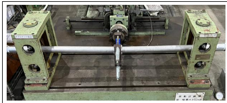
写真 4-21-1 耐震試験(震度 7 相当、加速度 947Gal)状態
