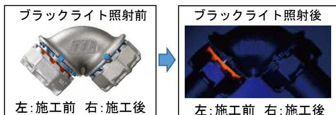
図 1-4 施工完了確認
