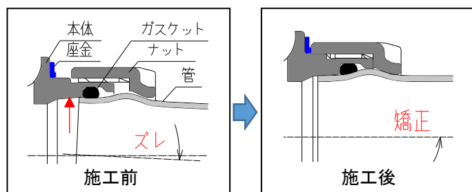
図 1-3 配管芯ズレ矯正
