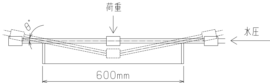
図 4-14 曲げ試験概略図
