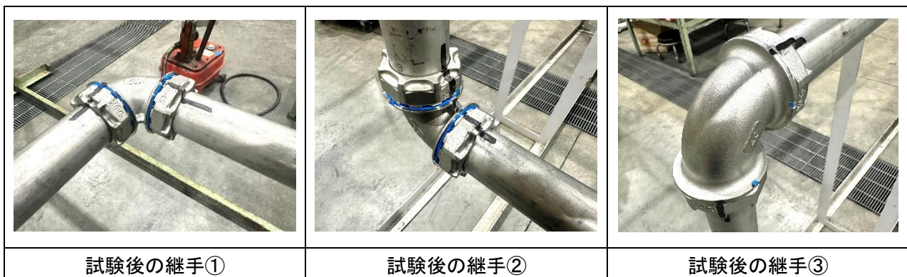
写真 4-16 揺動試験Ⅱ状態
