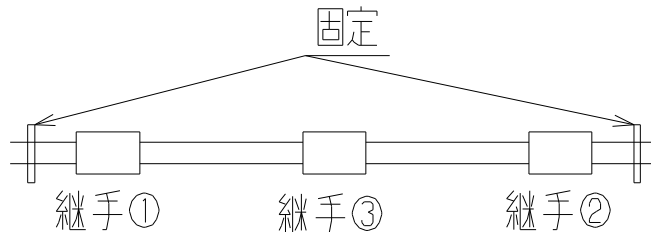
図 4-20 供回り試験概略図
