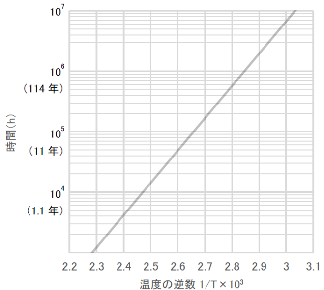
図 4-23 温度と寿命時間との関係
