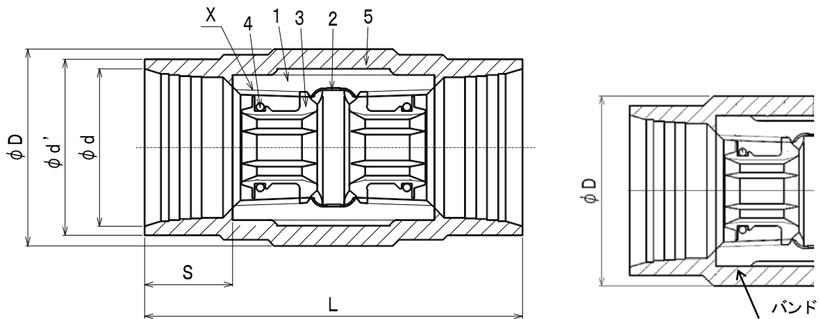
付図1. バンド有り製品の端部形状
