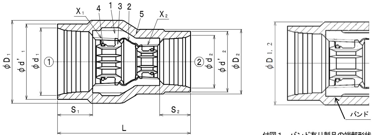
付図1. バンド有り製品の端部形状
